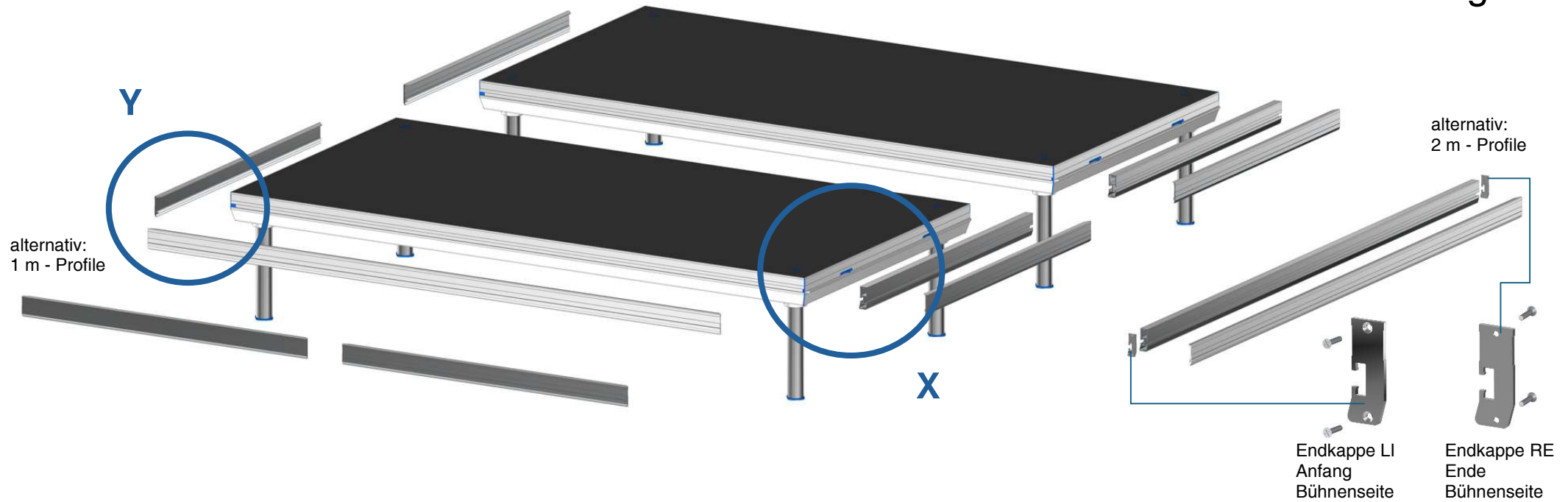
Ansicht Y
